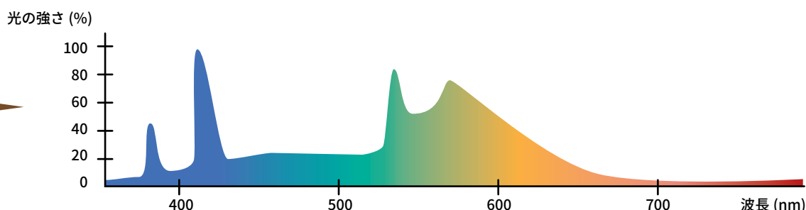
白色 蛍光灯 分光分布
