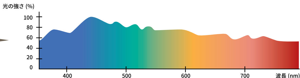
自然光 (昼光) 分光分布
